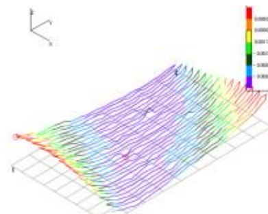
平面度測定 (ホワイトライトセンサ)
